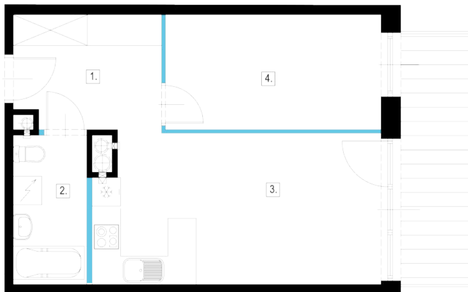
Rzut lokalu z zaznaczeniem jego położenia na kondygnacji
