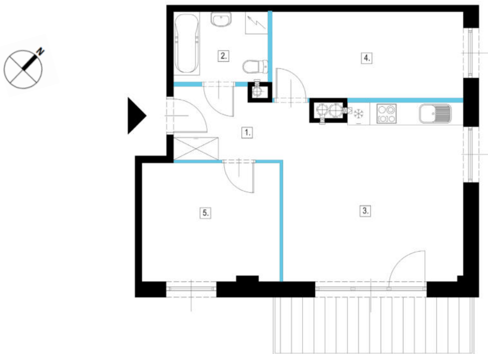
Rzut lokalu z zaznaczeniem jego położenia na kondygnacji
