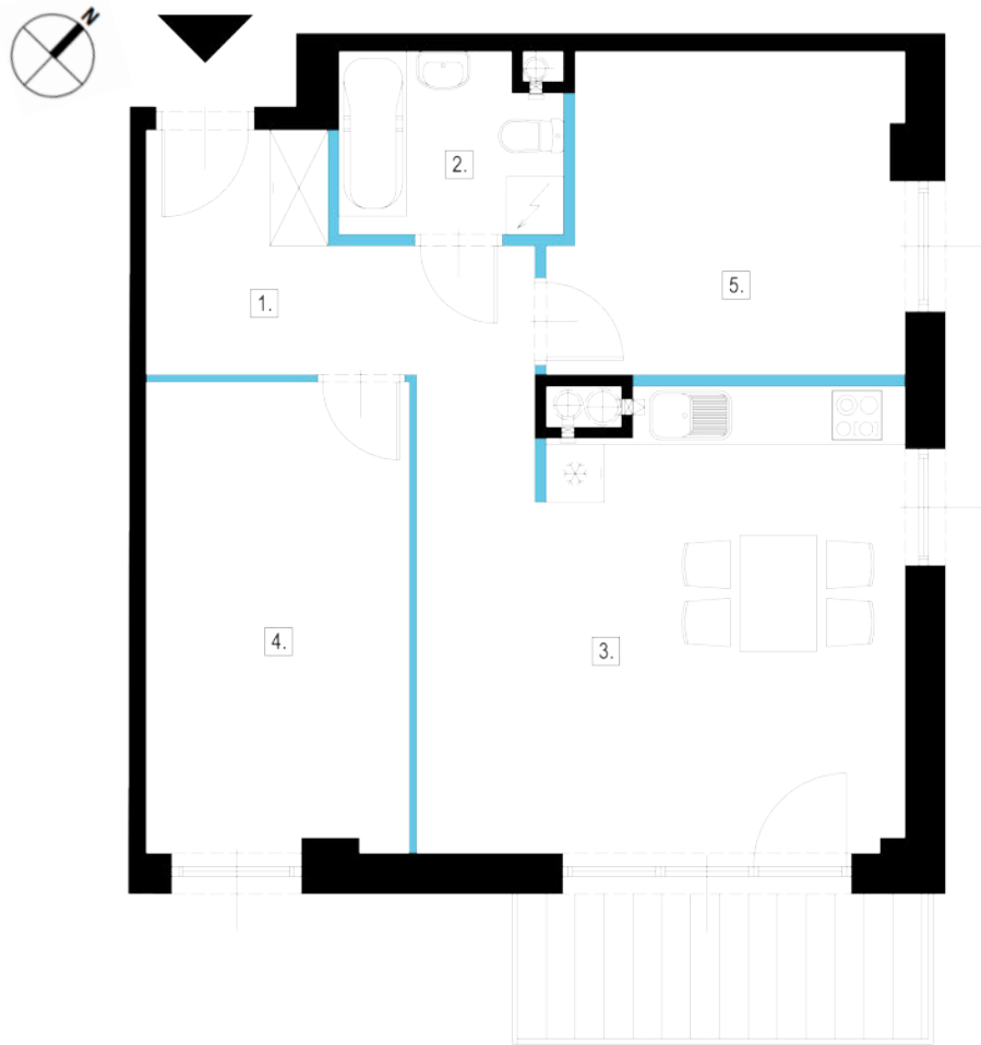
Rzut lokalu z zaznaczeniem jego położenia na kondygnacji
