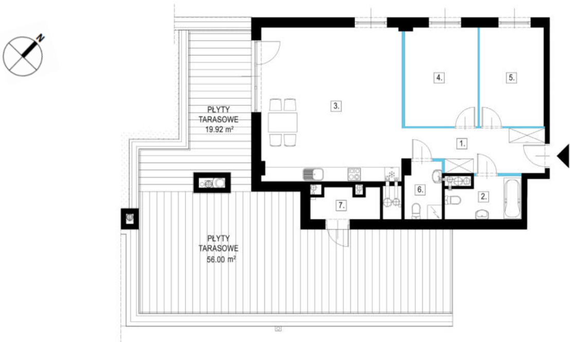
Rzut lokalu z zaznaczeniem jego położenia na kondygnacji
