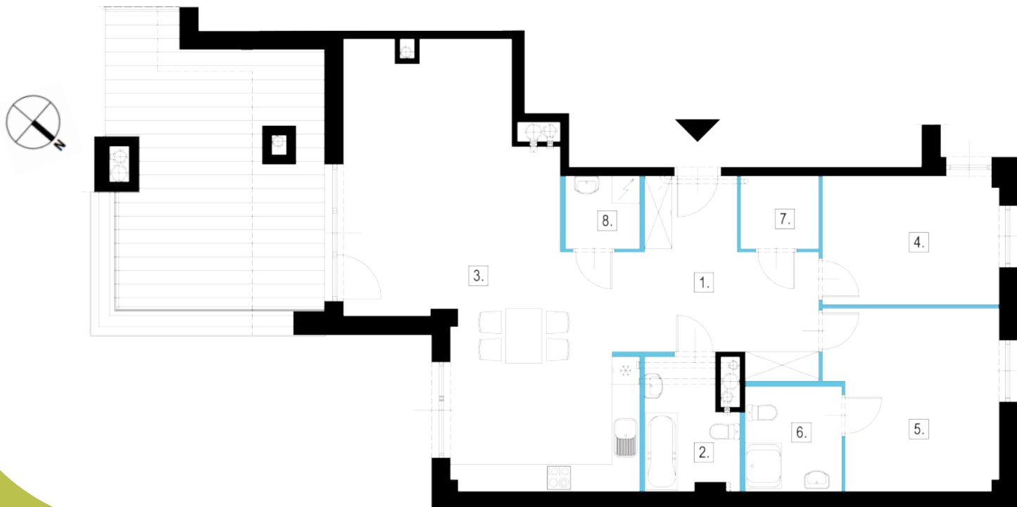
Rzut lokalu z zaznaczeniem jego położenia na kondygnacji
